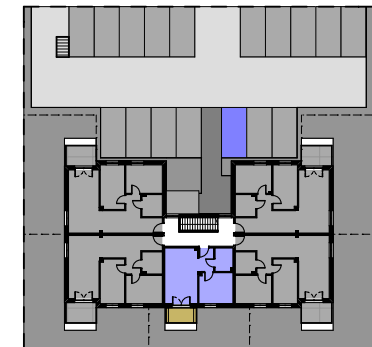
Widok kondygnacji
