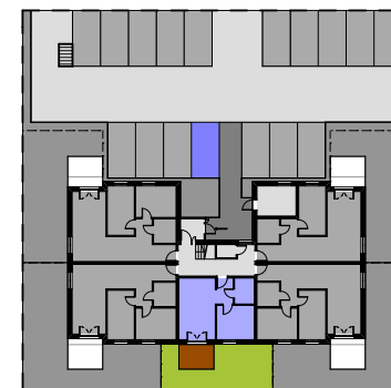
Widok kondygnacji
